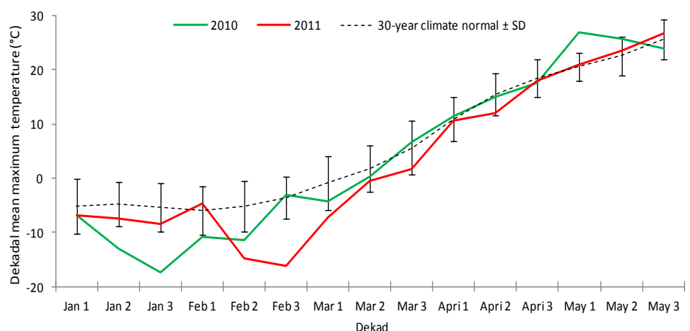
图 1. 俄罗斯 Aleksandrov-Gai 气象站（距离事发中心 80 km）记录的旬最高温平均值
