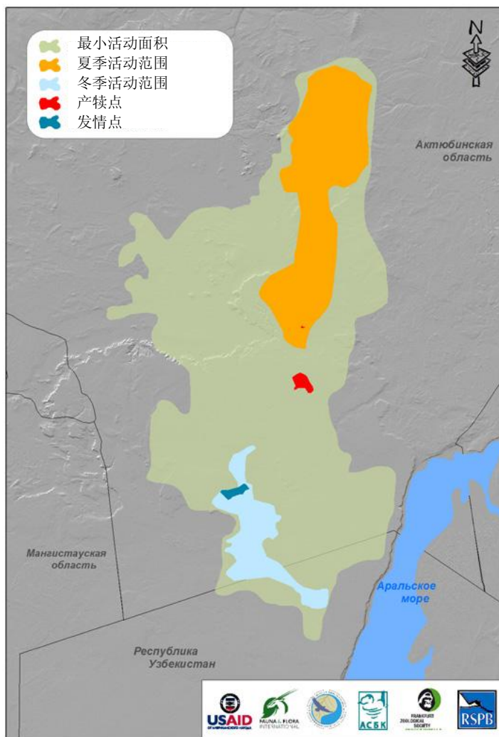
图 1. 使用最小凸多边形法获得的赛加羚羊年度活动范围及季节性活动范围。
